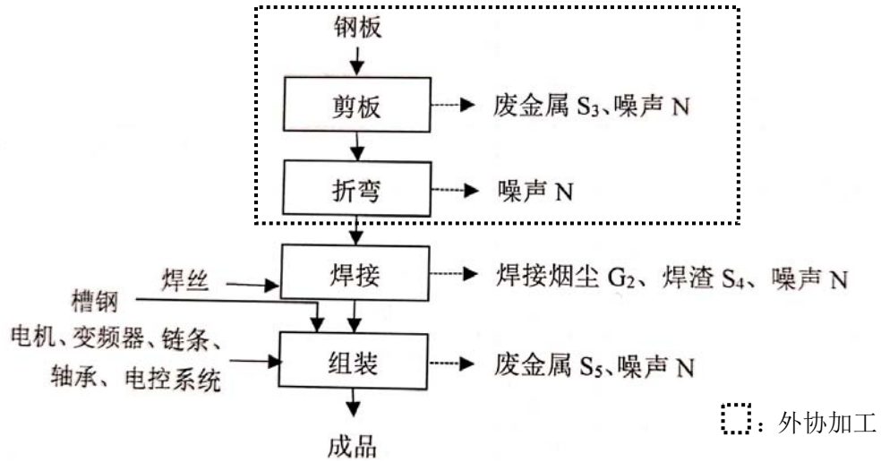
图 2-3 缠绕膜机生产工艺流程及产污环节图
